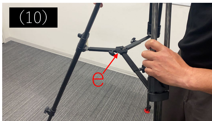
(10) 三脚の安定性を増すためにミドルスプレッダー)にあるネジeを緩めて、脚の支え部分をさらに伸ばします。
