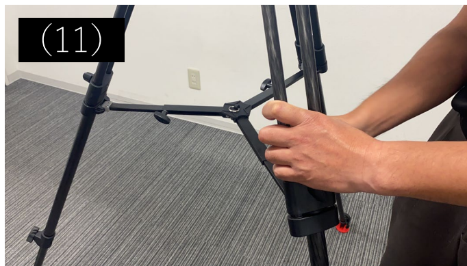
(11) 写真のように、全て伸ばしきって地面と平行になったことが確認できたら、カメラ三脚の準備は完了です。
