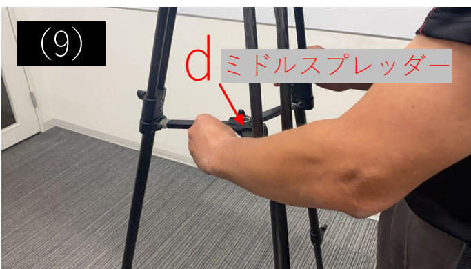
(9) 三脚がしっかり立つかどうかの確認と上記写真dのミドルスプレッダーの部分が地面と平行になっているか確認してください。
