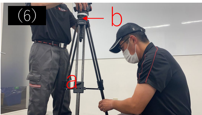
(6) b部分を最大に引き上げたら、aのネジ部分を締めます。
